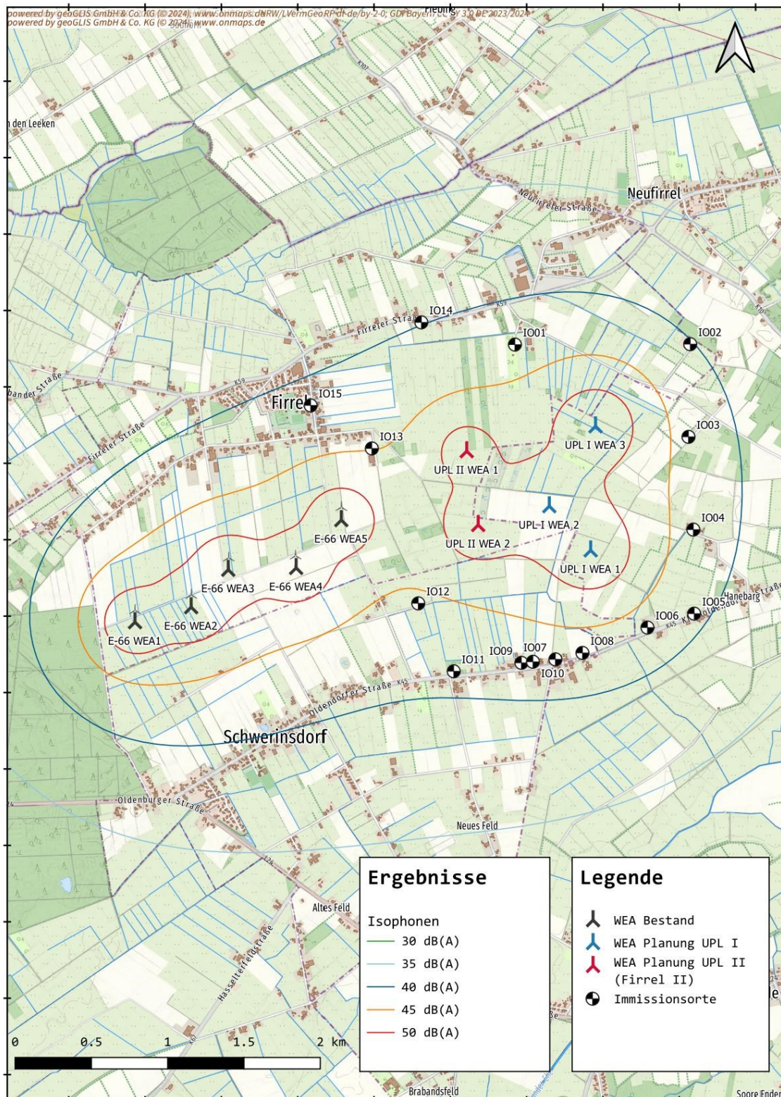
Abbildung 19: Isophonen der Geräuschbelastung durch die bestehenden und den geplanten WEA für den Betrieb im Nachtzeitraum an den maßgeblichen Immissionsorten im Sinne der TA Lärm [1].
