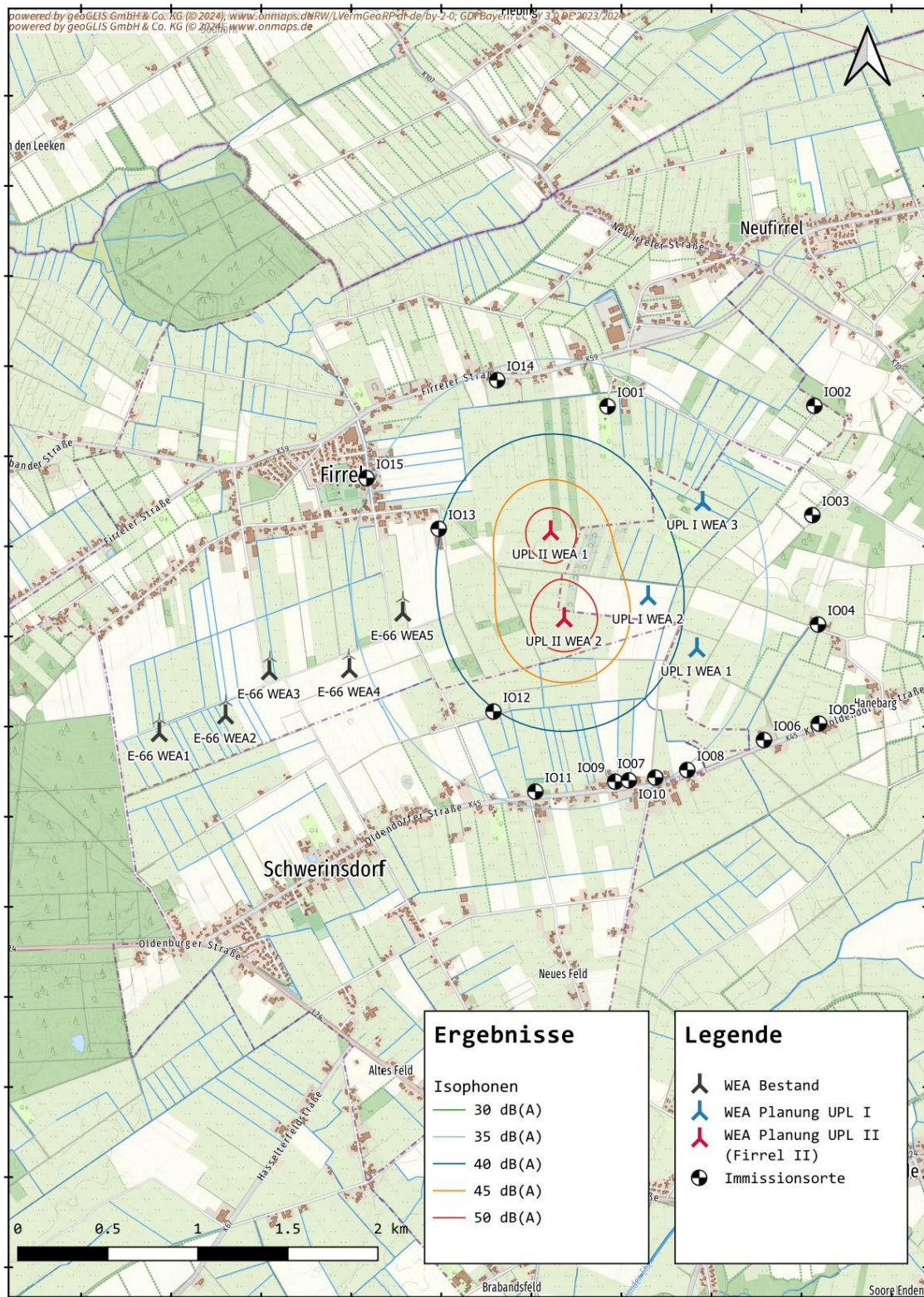
Abbildung 18: Isophonen der Geräuschbelastung durch die geplanten WEA für den Betrieb im Nachtzeitraum an den maßgeblichen Immissionsorten im Sinne der TA Lärm [1].
